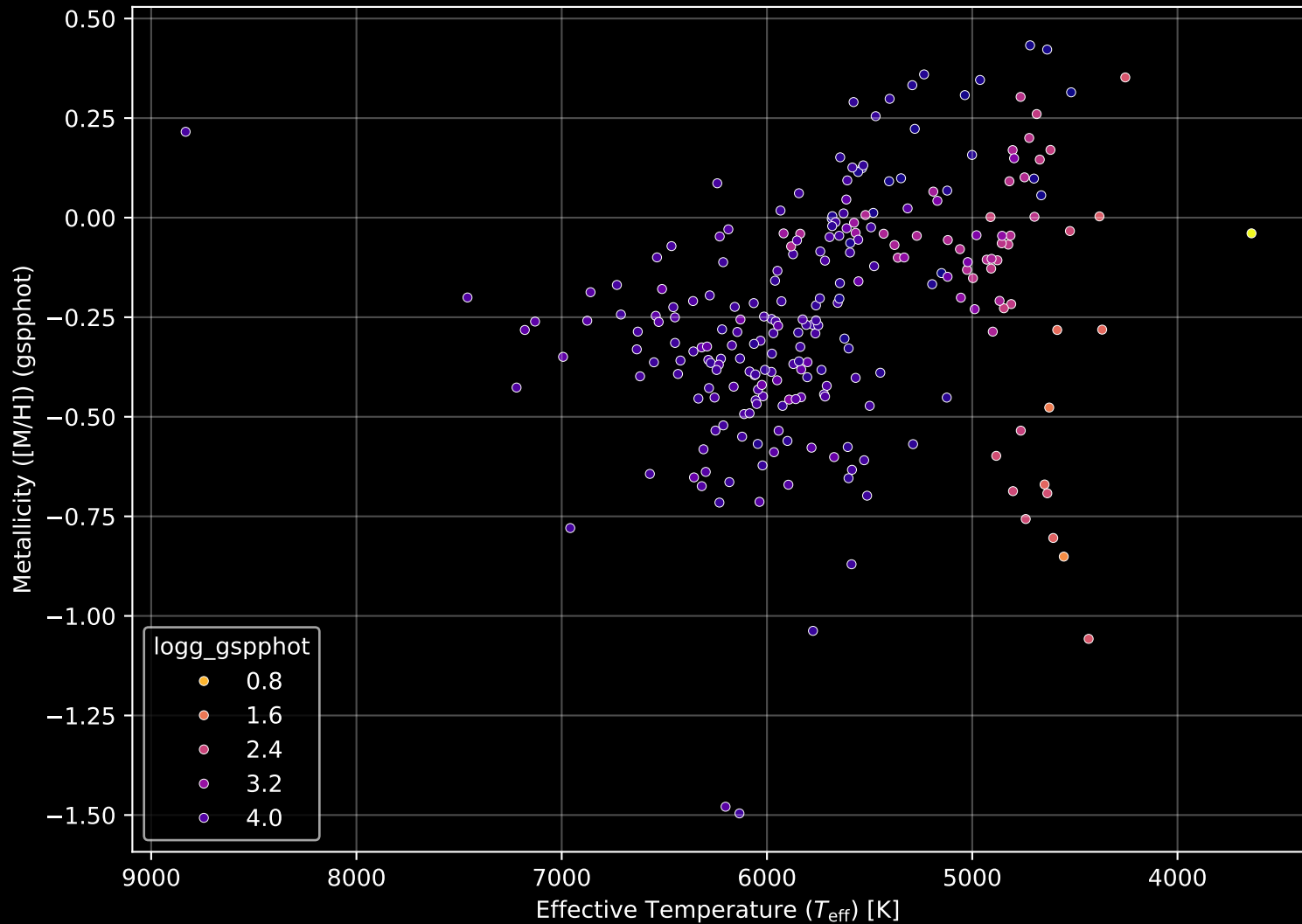
GALAH DR4 Field: [7149] Stellar Population Parameters (n= 244)
