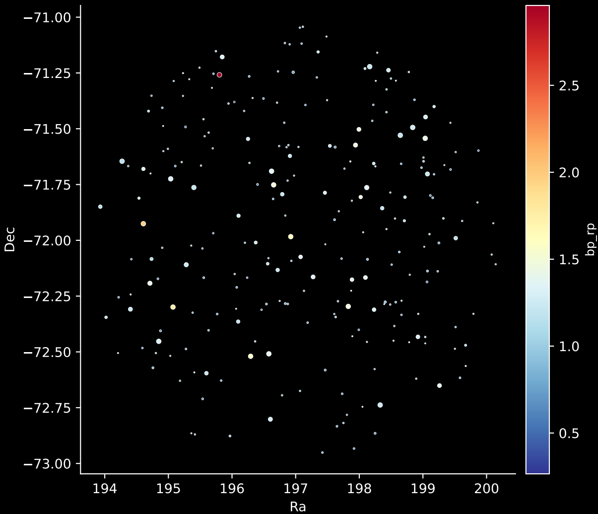
GALAH DR4 Field: [7149] Stars: 244
