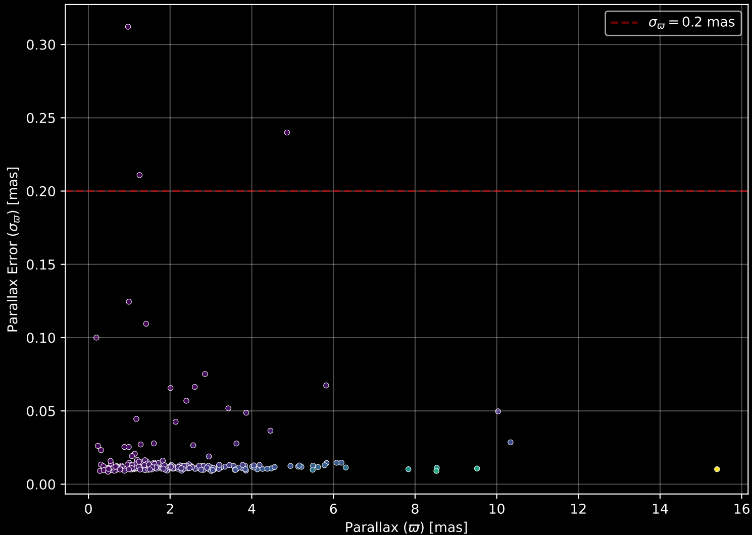
GALAH DR4 Field: [7149] Parallax Quality (n= 244)
