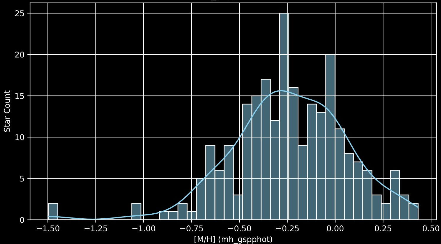
GALAH DR4 Field: [7149] [M/H] (mh_gspphot) (n= 244)
